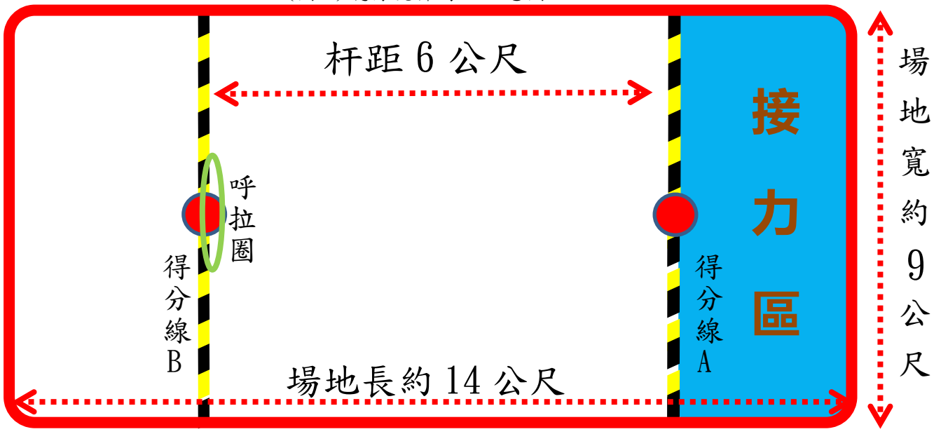
(圖 3) 飛行繞杆場地示意圖
