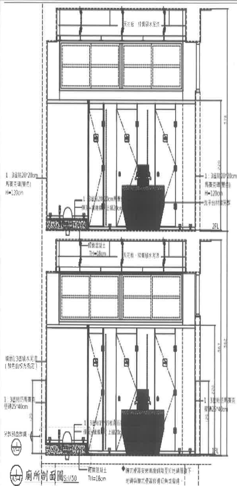
二樓女廁磁磚計畫示意圖 S3730
