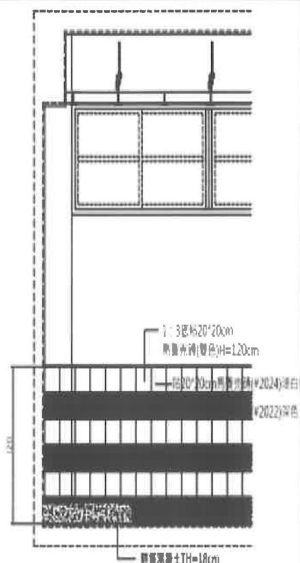
二樓女廁磁磚計畫示意圖 S3730
