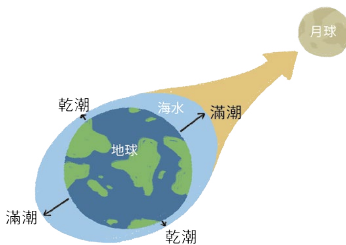
圖25. 潮汐示意圖
