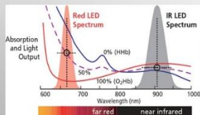
血氧濃度計偵測原理
